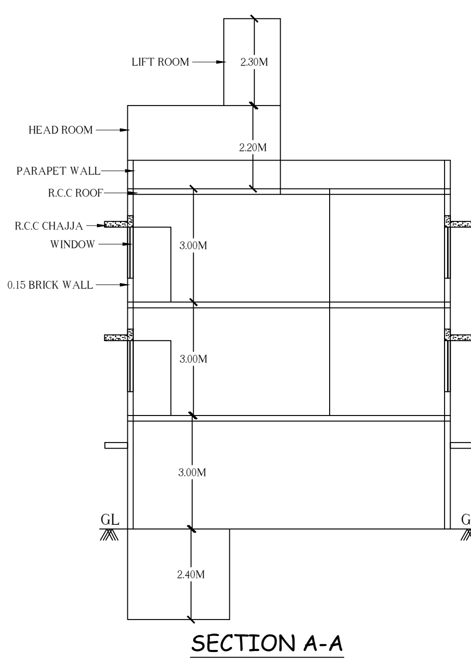
SECTION A-A
